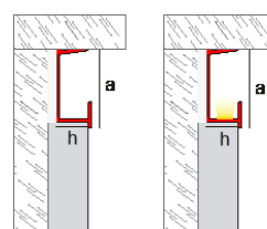
Couronnement supérieur
