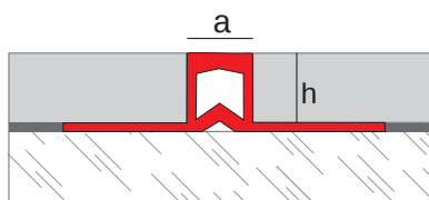
Novojunta® 2 PVC
