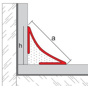
Novoescocia® 4 alluminio
