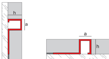
Novolistel® 3 alluminio
