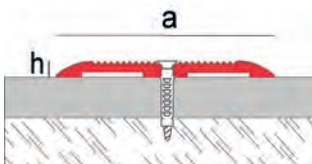
Novopletina® alluminio
