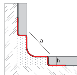
Angle intérieur
