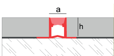
Novojunta® 3 PVC
