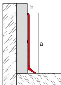
Novorodapie® L
