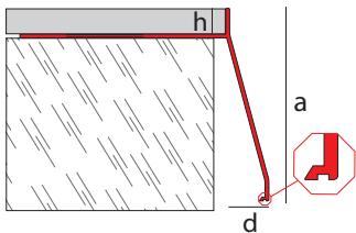
Novovierteaguas GT
