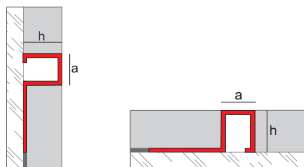
Novolistel® 3 aluminium
