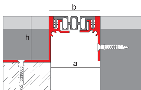
Version périmètre
