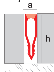
Novojunta® 1 PVC
